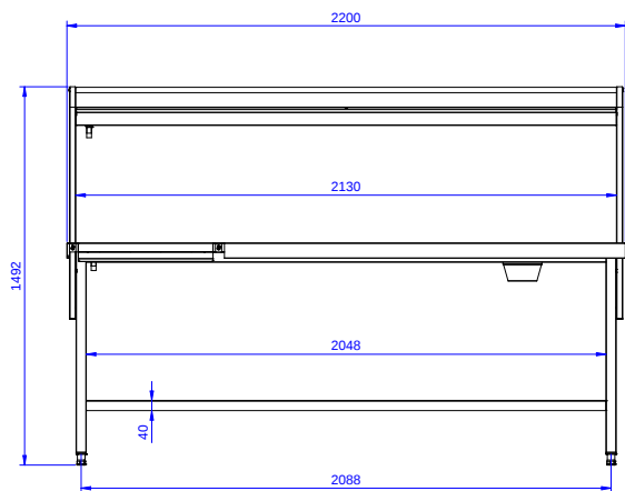
Boční
